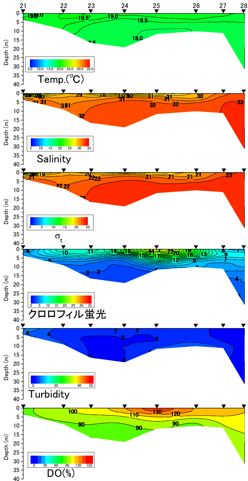
有明海東ラインの水温(°C)、塩分、密度( \sigma_t )、クロロフィル蛍光強度、濁度、溶存酸素飽和度(DO%)の鉛直面図(国土交通省の調査による) (2017年5月16日)
